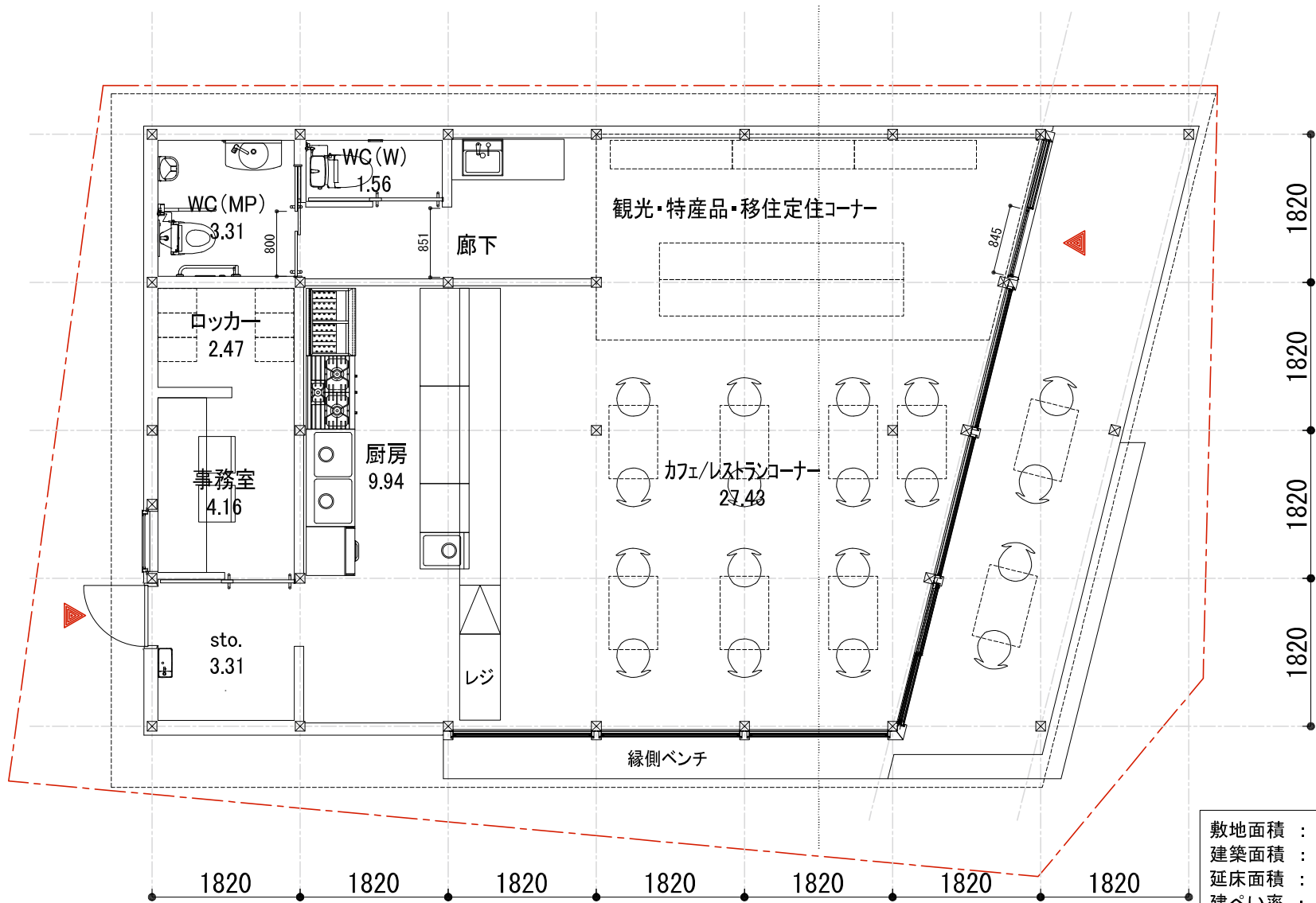
平面図 <1 : 50>
